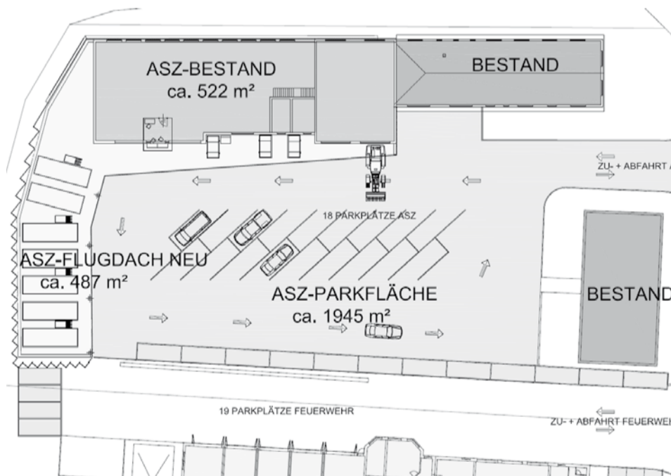
So sieht der Planungsentwurf von Michael Haderer zum Altstoffsammelzentrum Pregarten aus.
